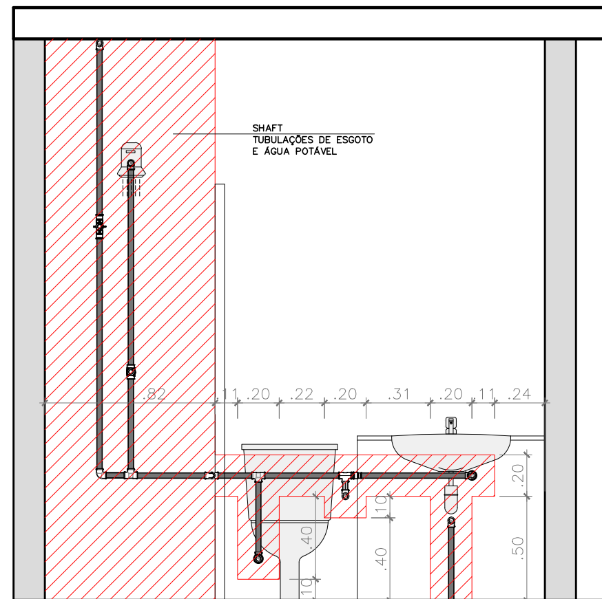
VISTA A ESC._1/25
